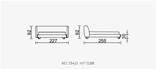
Bon Bon Bedstead (180)
